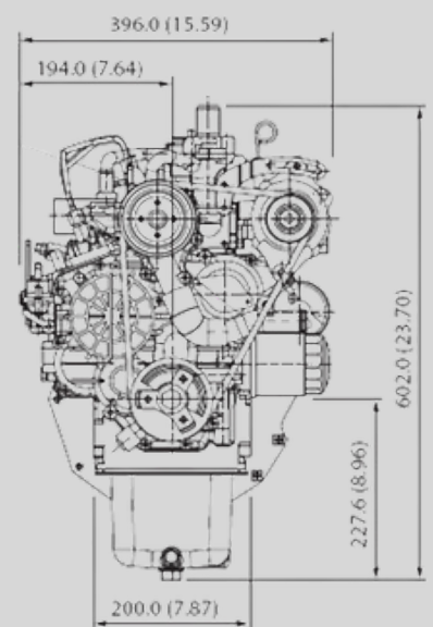
KUBOTA D1105
