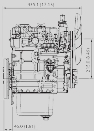
KUBOTA D722
