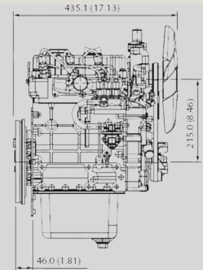
KUBOTA D722
